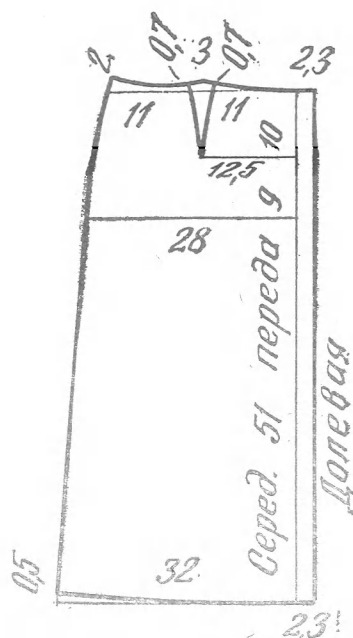
Переднее полотно юбки - 2 дет. (Мод. 1)
